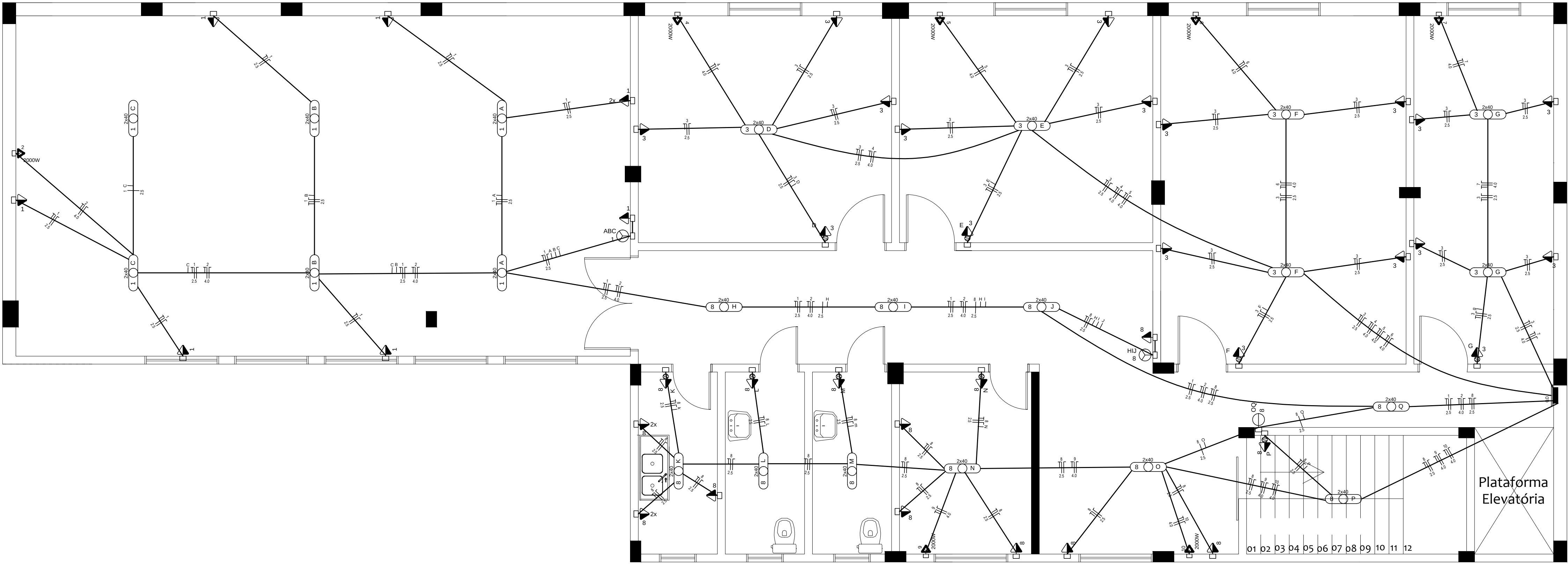
PLANTA BAIXA- ELÉTRICO - PAV SUPERIOR ESC: 1/50
