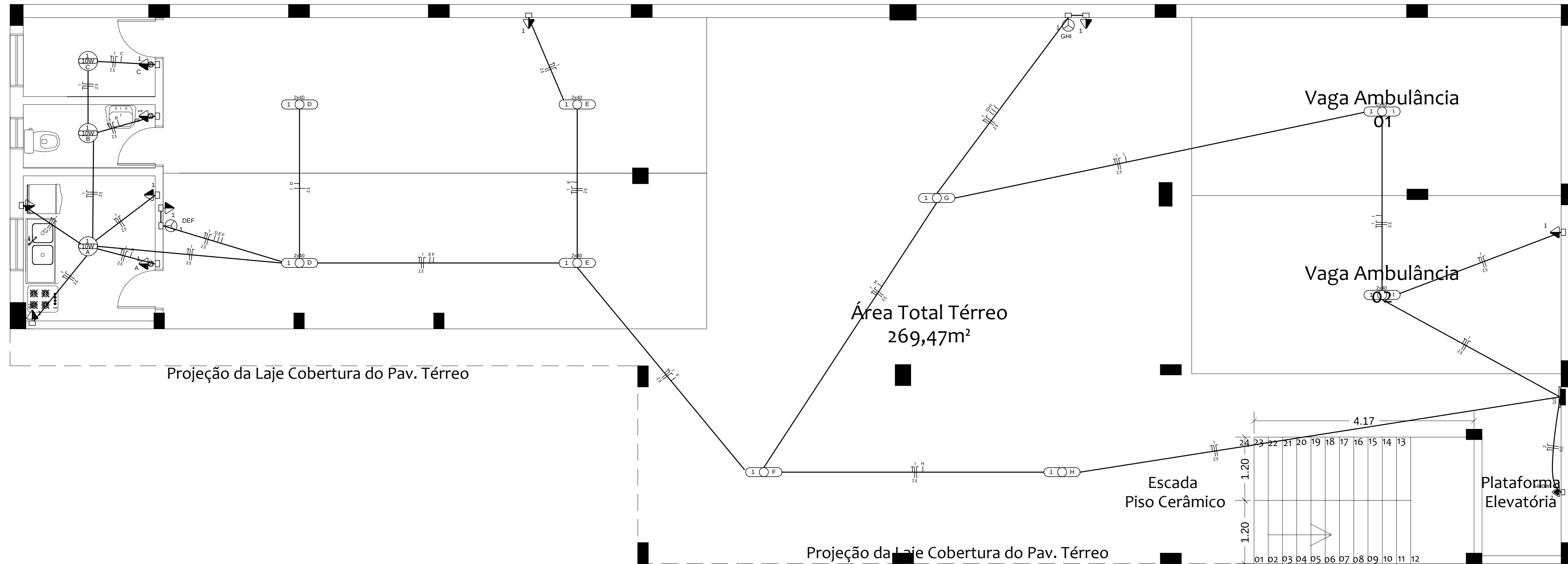
PLANTA BAIXA- ELÉTRICO - PAV. TÉRREO ESC: 1/50
