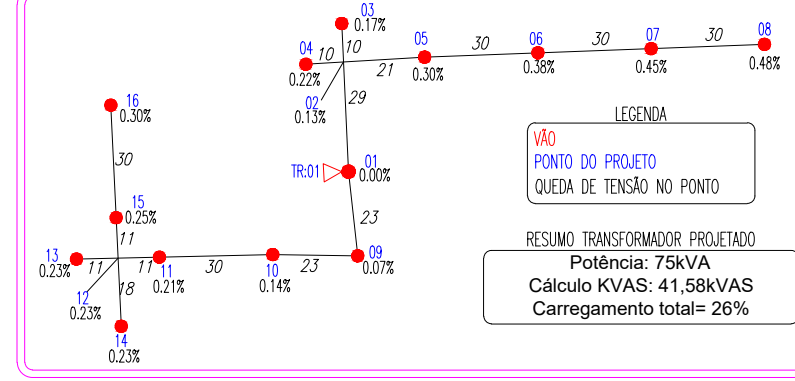
DIAGRAMA UNIFILAR DA REDE SECUNDÁRIA
