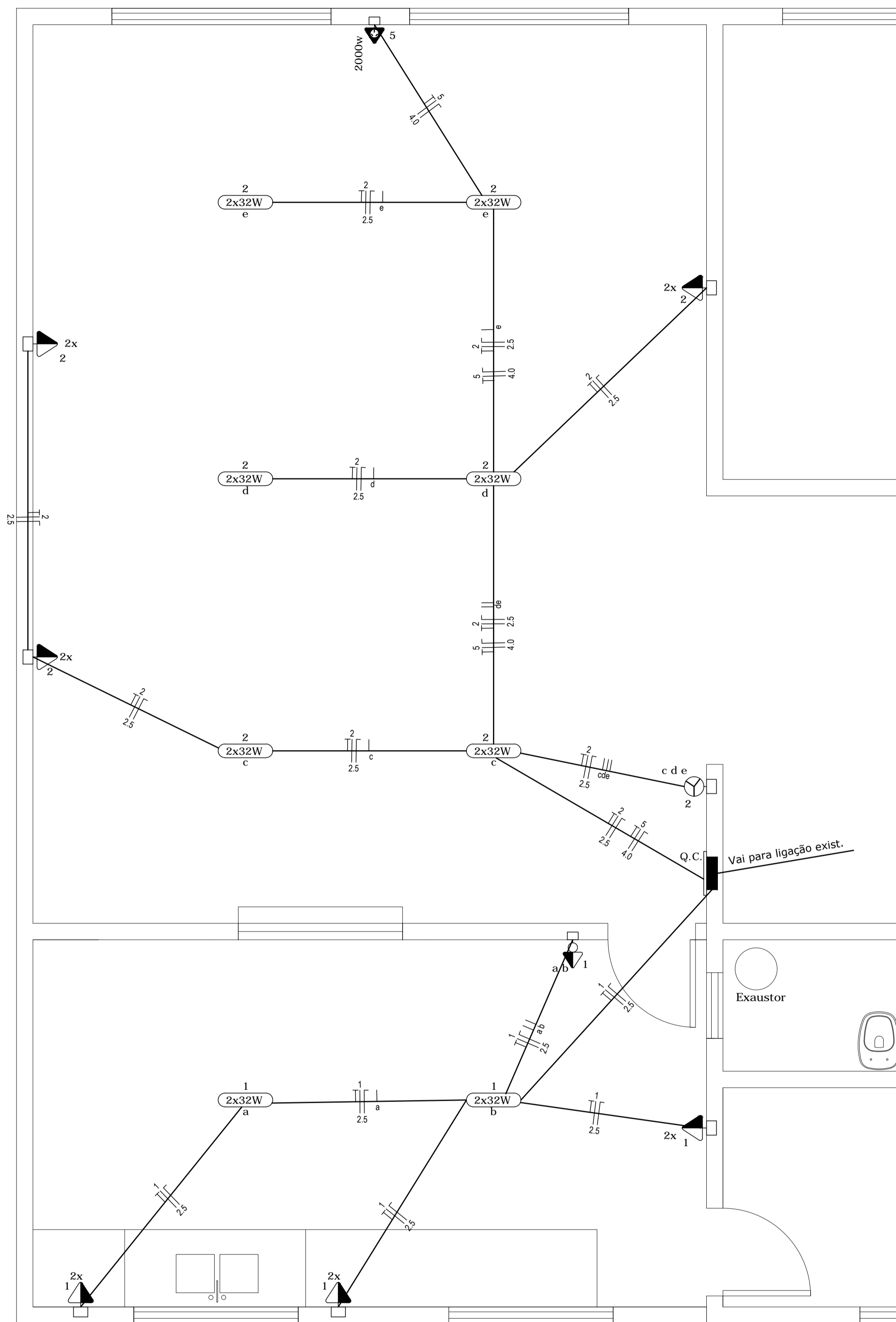
PLANTA BAIXA - ELÉTRICO ESC: 1/50
