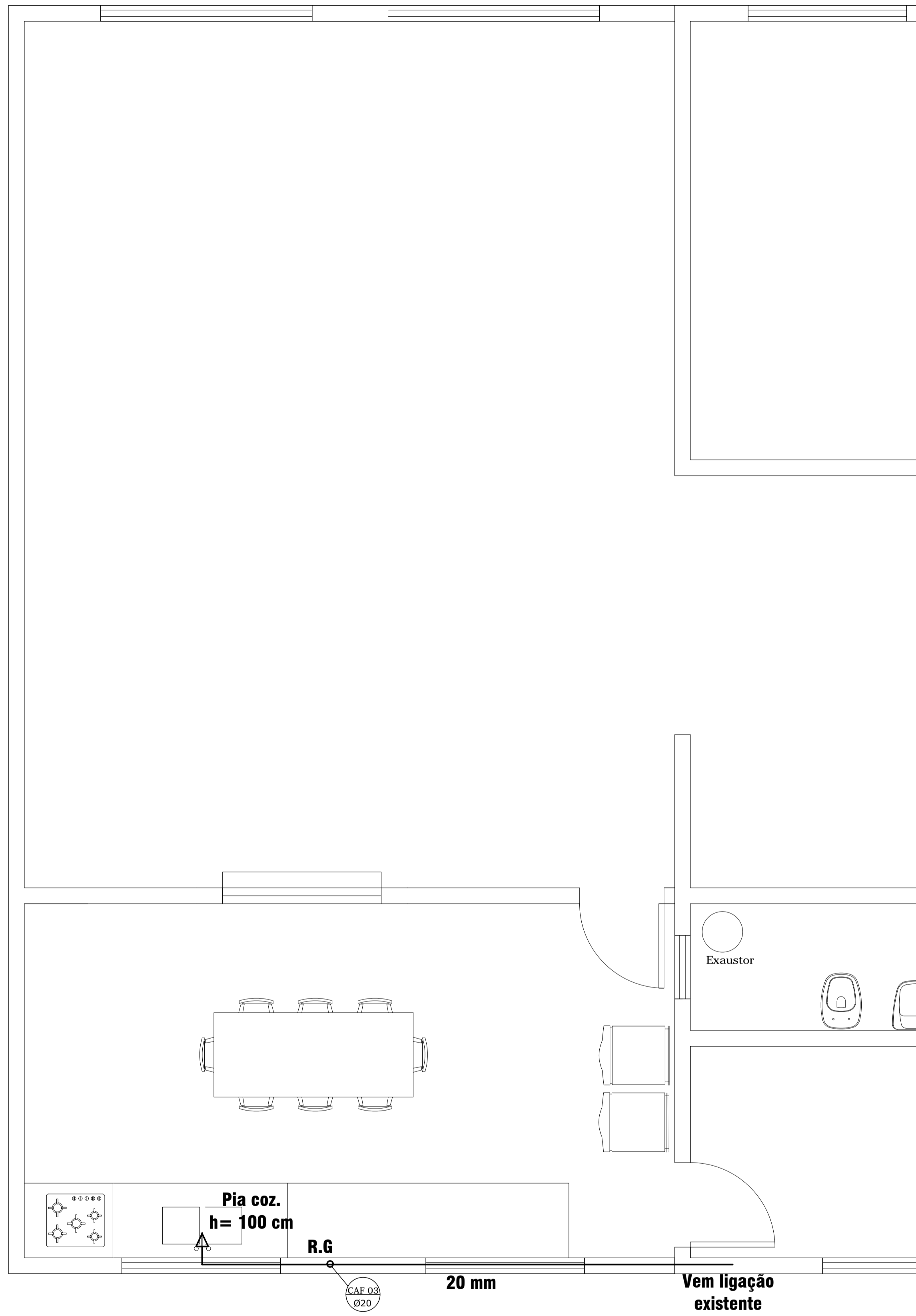
PLANTA BAIXA - ÁGUA FRIA ESC: 1/50
