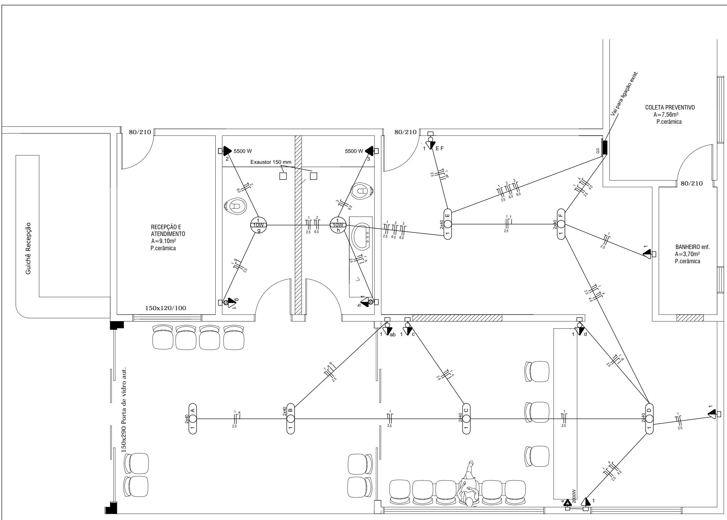
PLANTA BAIXA ELÉTRICO - TÉRREO A: 58,26 m 2
