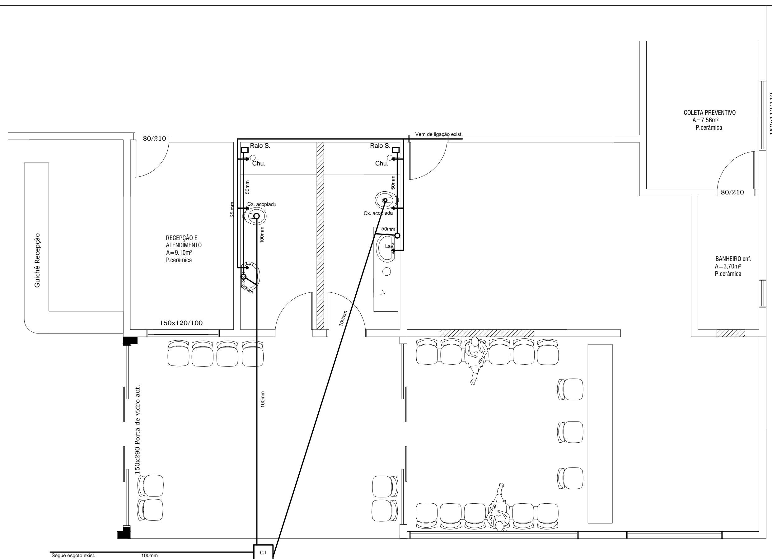
PLANTA BAIXA HIDROSSANITÁRIO - TÉRREO A: 58,26 m 2
