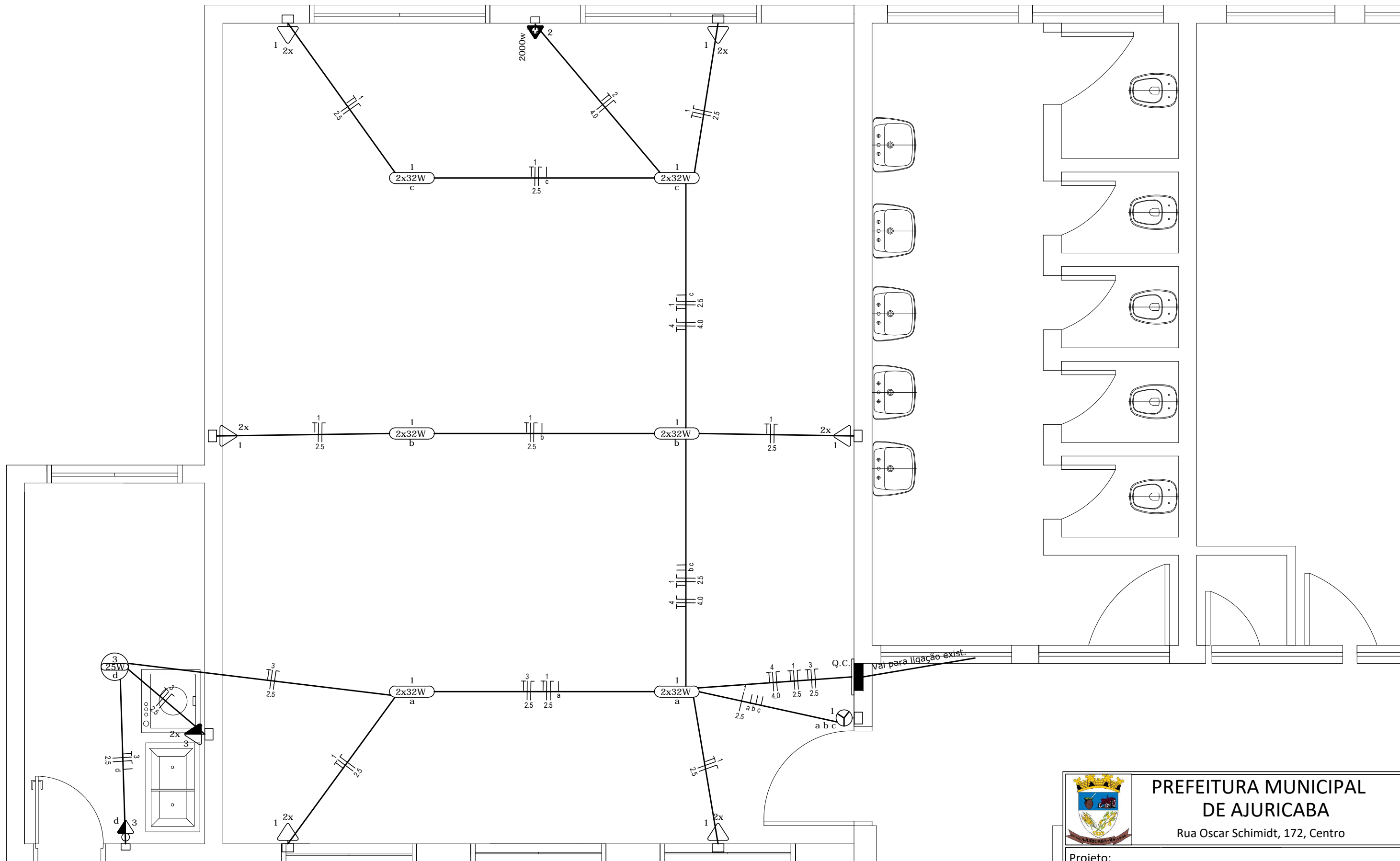
PLANTA BAIXA - ELÉTRICO ESC: 1/50
